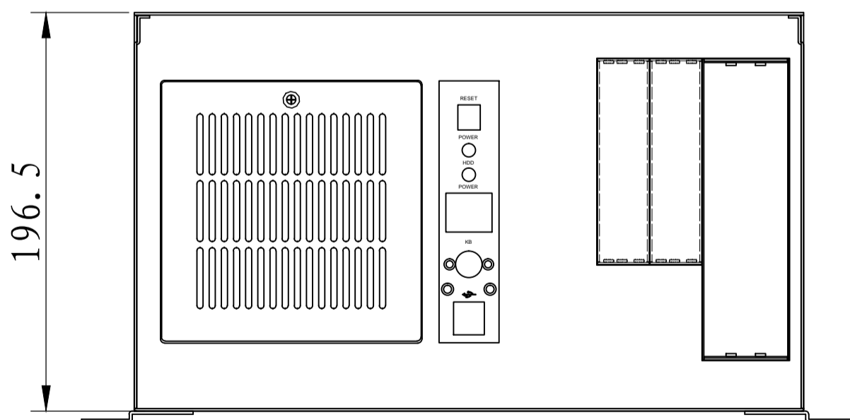
P向视图
